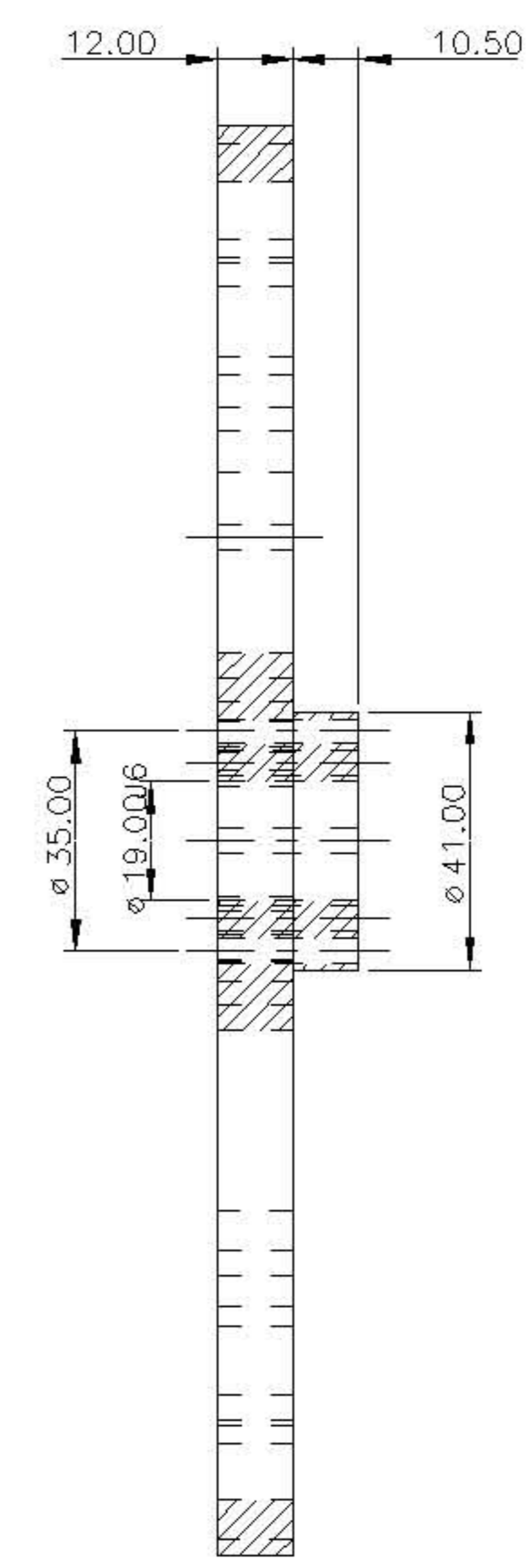
SECTION A-A
